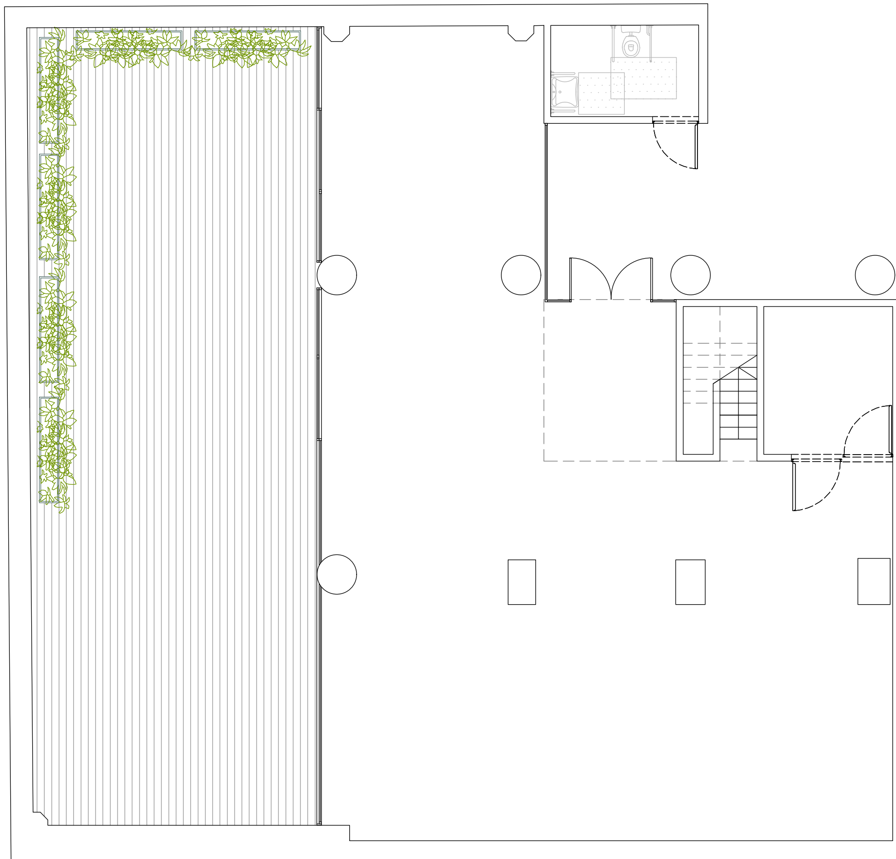
PLANTA BAJA
